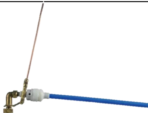
4720/21 FLOTANTE INTERCAMBIABLE H.A CODO FLUMAX
