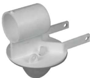
4700/33 FLAPPER CON VASO PLASTICO COMPLETO
